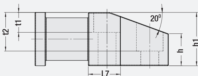
Die Lifting Lug
